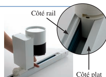
c) Mettre le spot sur le rail : attention au sens.
