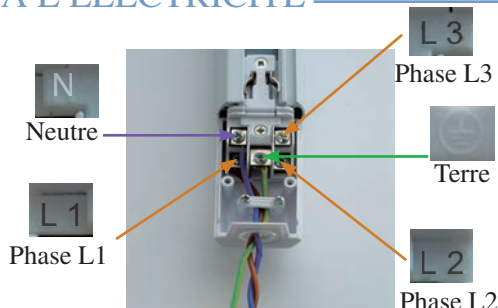
b) Relier les fils de votre câble préalablement dénudé comme sur la photo ci-dessus, et sélectionnez une des 3 phases ( L1, L2, L3)
